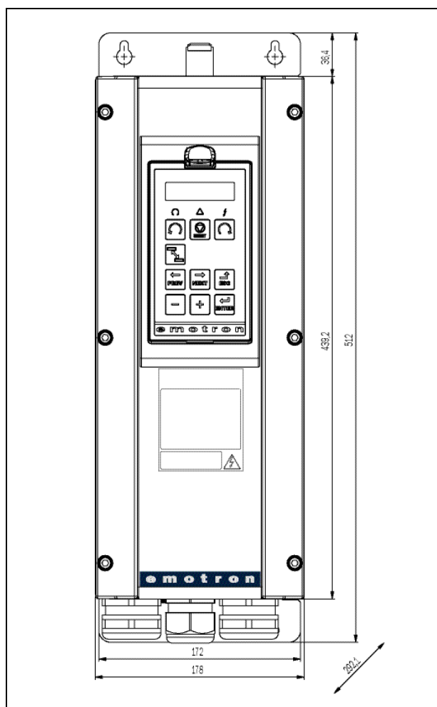
Fig. 2 FDU48/52: Modelos de variador 026 a 046 (C)
