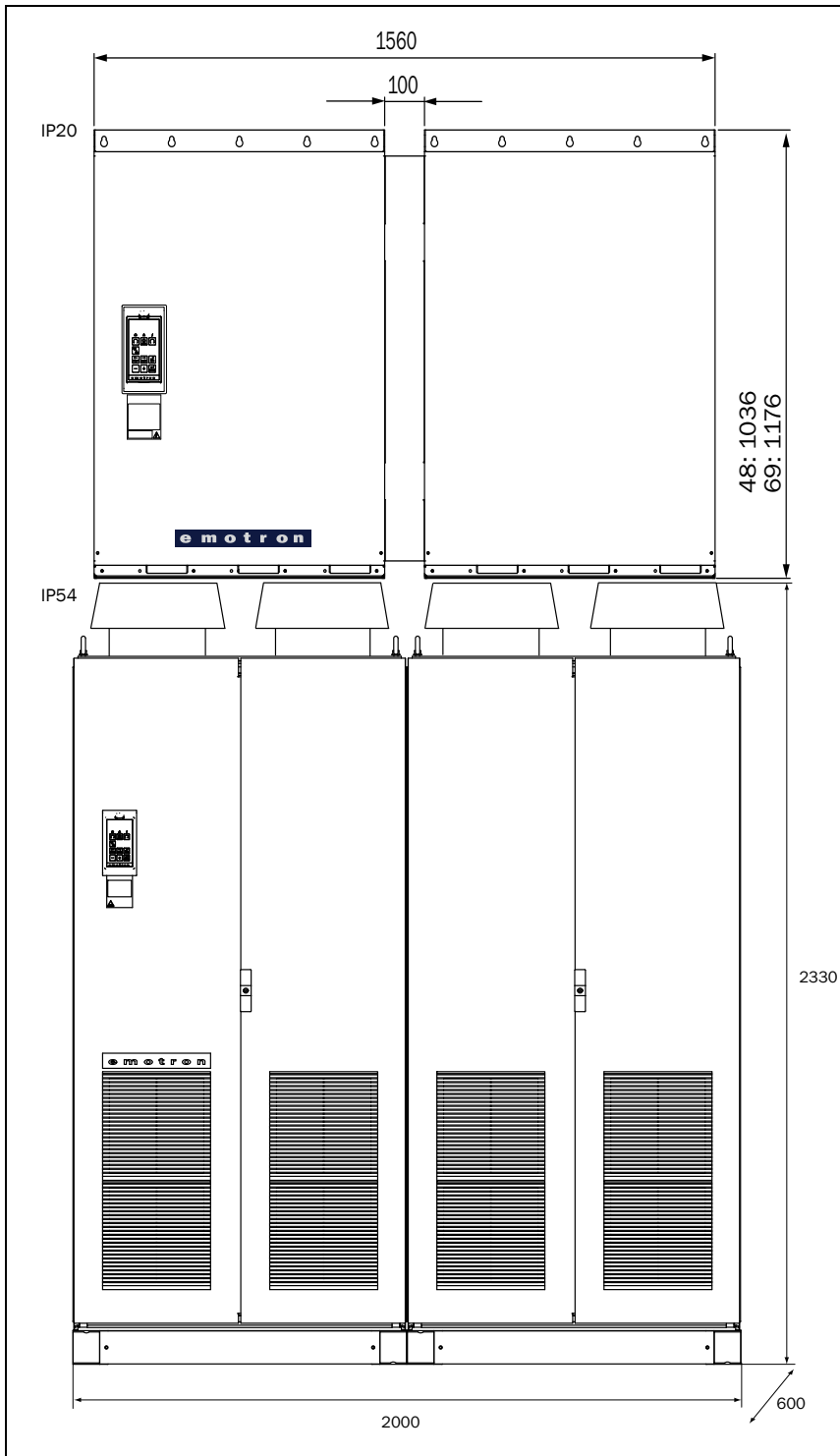
Fig. 9 FDU48: Modelos de variador 1200 a 1500 (K) FDU69: Modelos de variador 750 a 1000 (K69)
